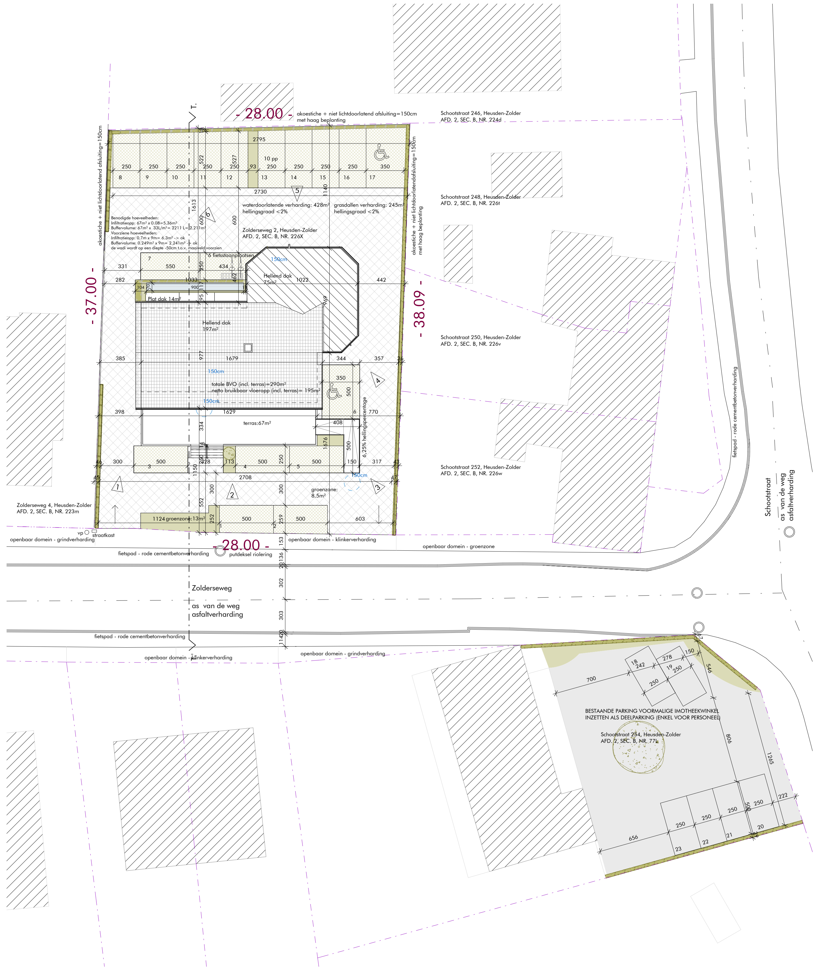
Inplantingsplan - nieuwe toestand 1 : 200
