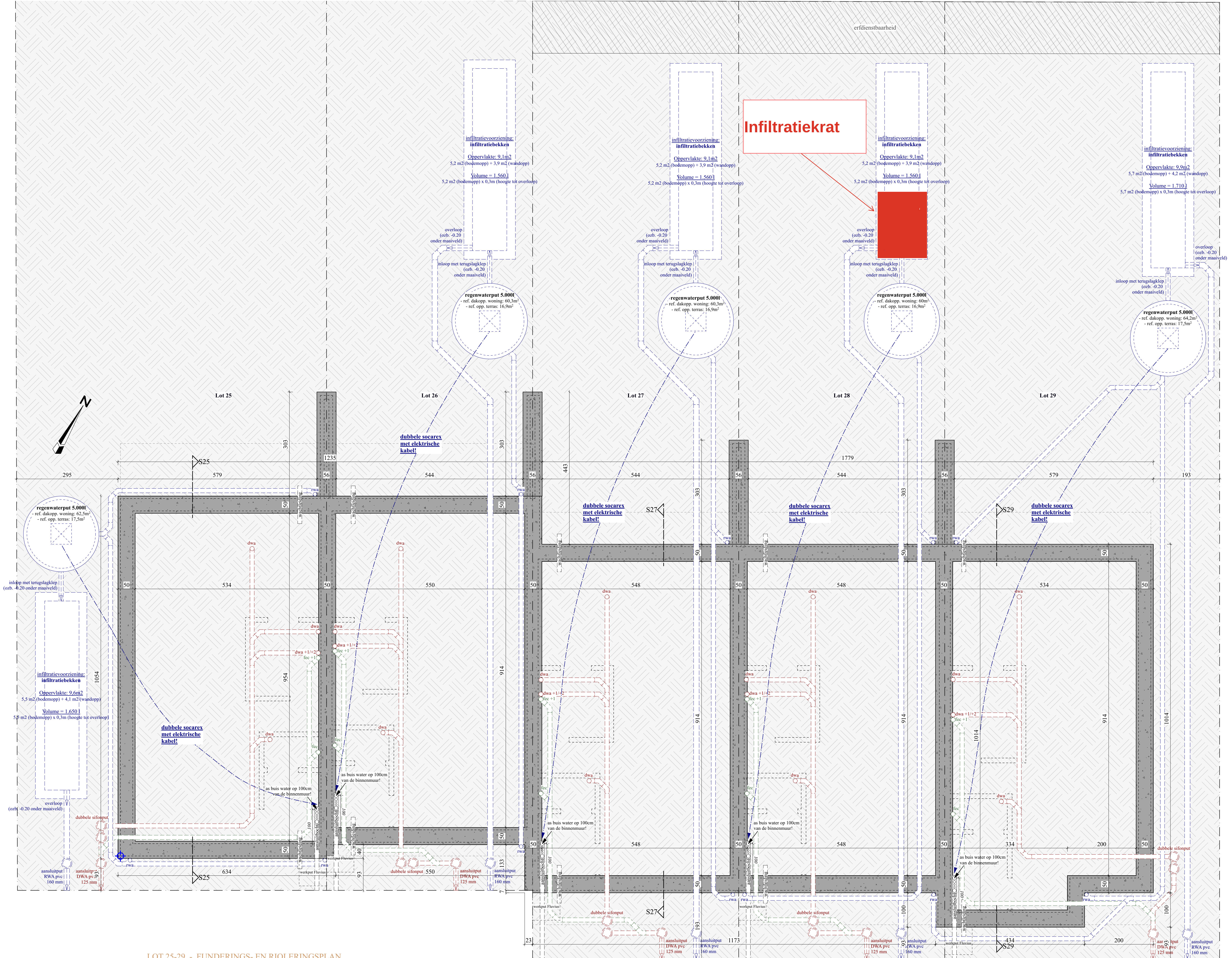
LOT 25-29 - FUNDERINGS- EN RIOLERINGSPLAN
