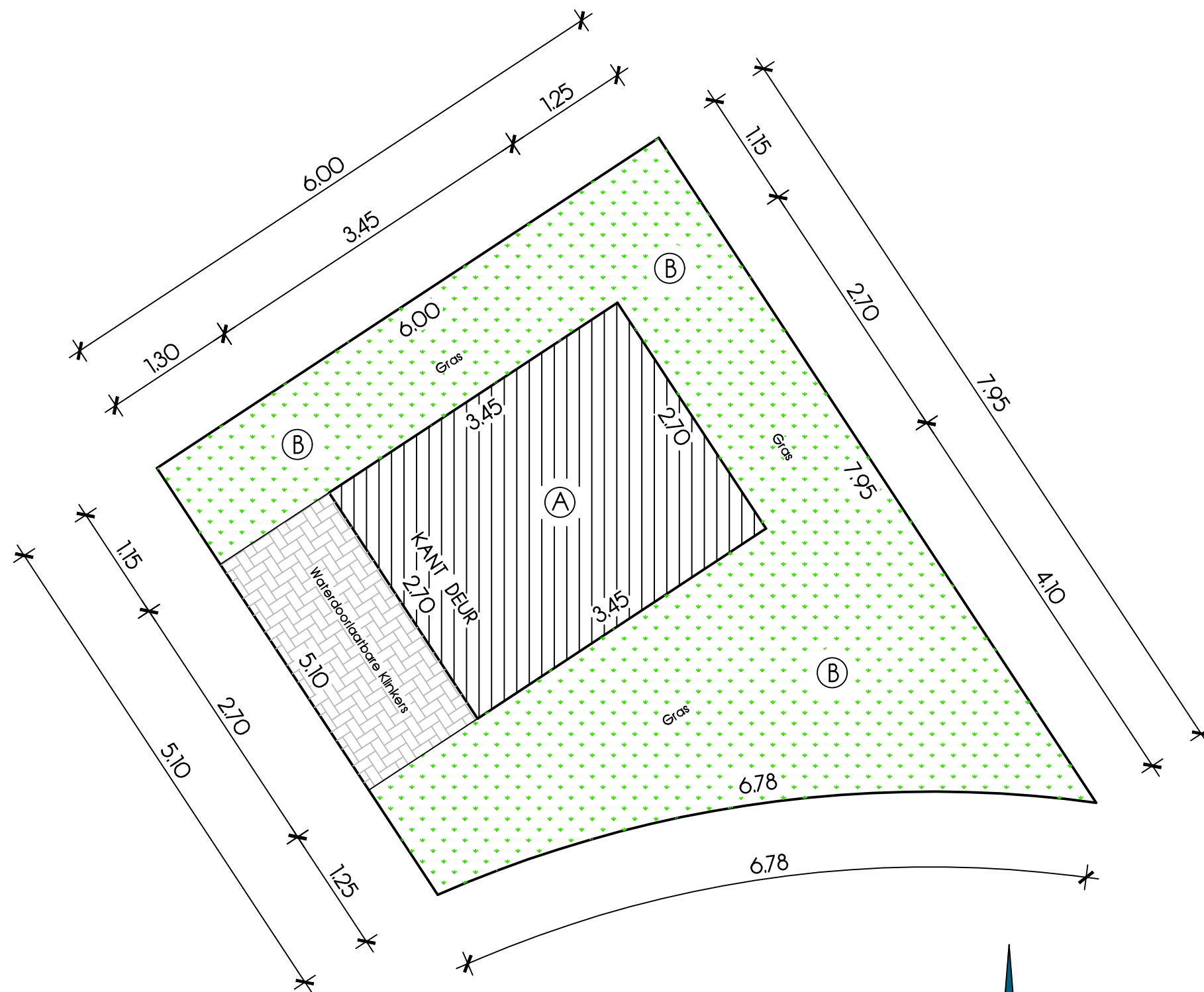
DETAIL PERCEEL GROND & HS-CABINE OP SCHAAAL 1 / 50
